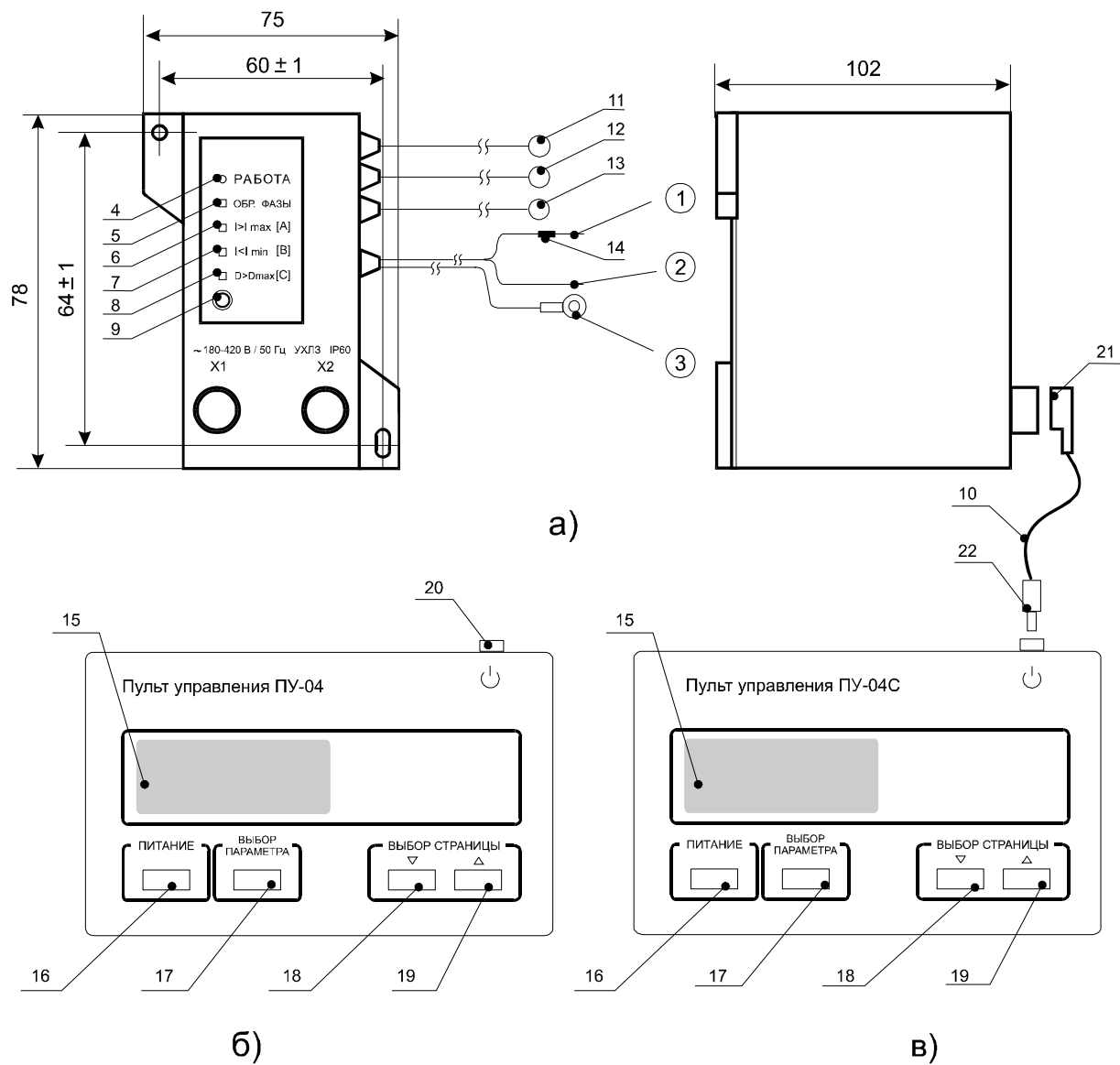
Рис.1. Внешний вид реле
