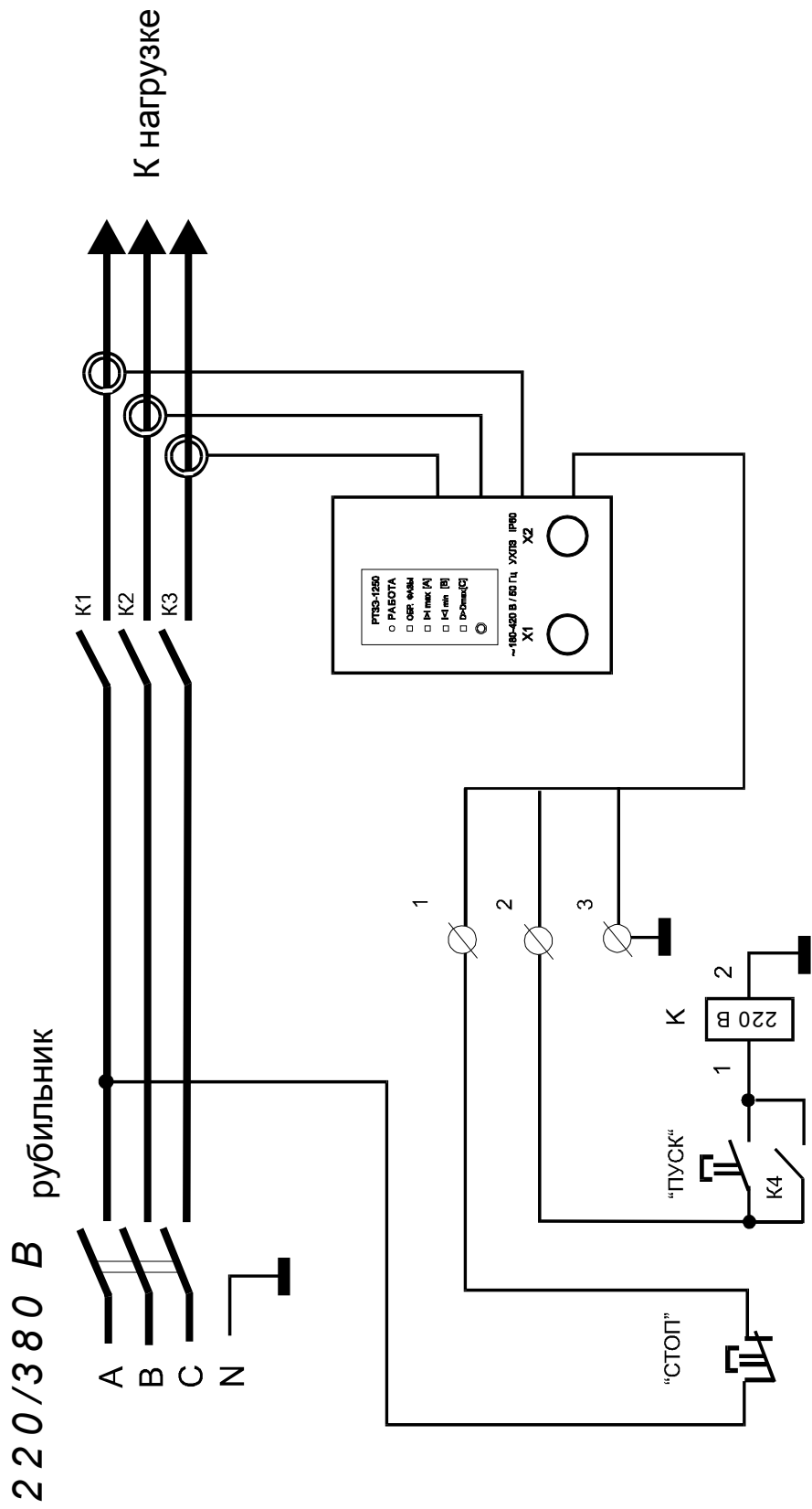
Рис.3.Подключение реле в схему управления контактора с предотвращением самозапуска при восстановлении питания (вариант 2)
